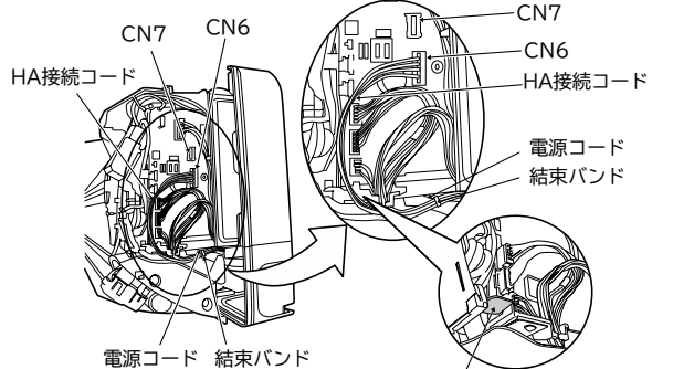
電源コード 結束バンド 上図はHAシステム (CN6) 接続時 ペンチ等で切り取り、あいたスペースにHA接続コードをはわせてください。
