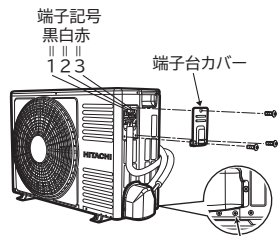
アース端子
