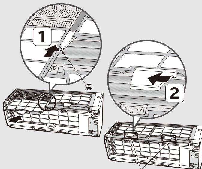
上面フィルターロック
