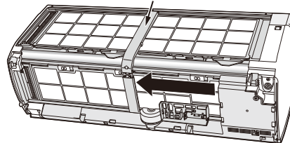
フィルター掃除ユニット
