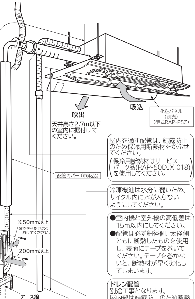
室内・室外機据付図(平地置台設置例)
