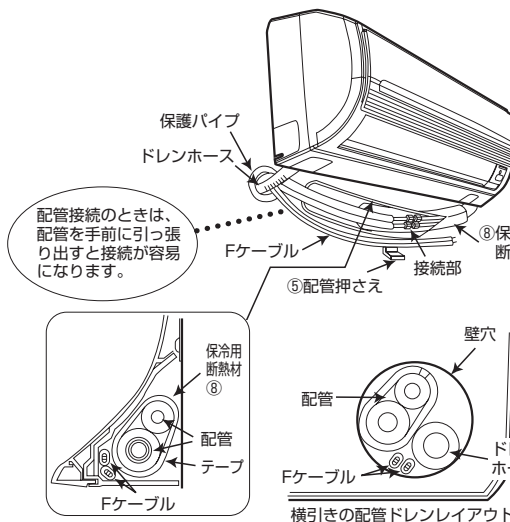
横引きの配管ドレンレイアウト
