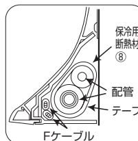
横引きの配管ドレンレイアウト
