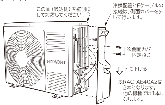
RAC-AE28A・AE40A2
