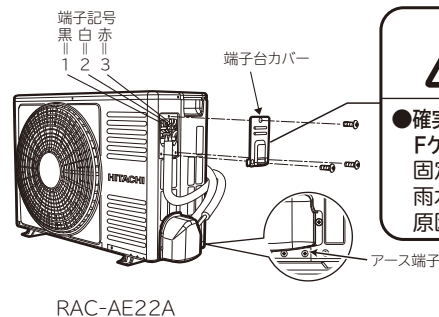
RAC-AE22A
