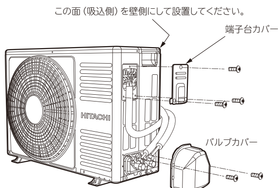
RAC-AE22A
