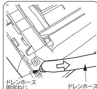
ドレンホースの外しかた
