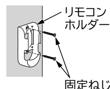
固定ねじ
