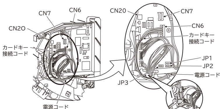
上図はカードキー (CN6) 接続時の例
