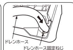
②ドレンホースは、固定ねじの穴をあわせて突き当たるところまで確実に押し込み、②で外した固定ねじで固定してください。
