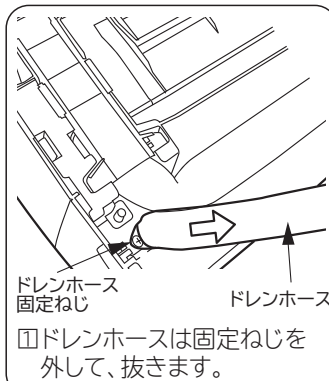
ドレンホースの外しかた
