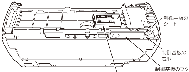
無線LAN接続アダプター
