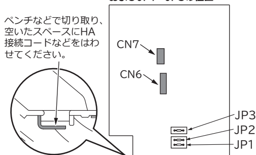
基板上のCN6・CN7の位置 およびJP1～JP3の位置
