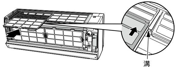
上面フィルターロック
