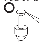
真円で均一に フレア加工され ていること。
