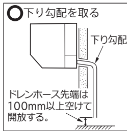
ドレン配管(VP-20)
