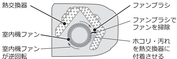
室内機断面図（イメージ）
