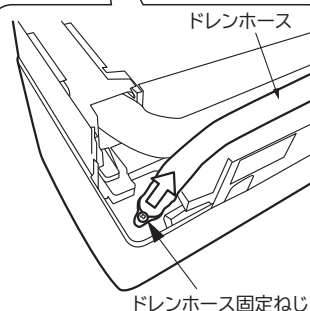
ドレンホース固定ねじ
