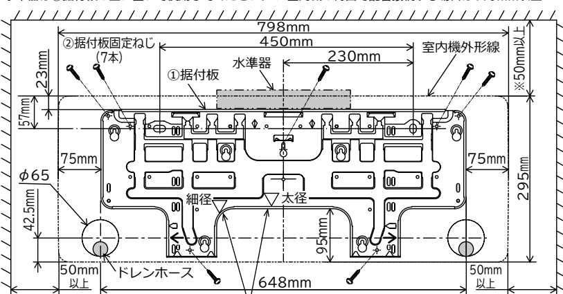
左引き出し時、室外機からの冷媒配管位置
