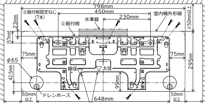
左引き出し時、室外機からの冷媒配管位置
