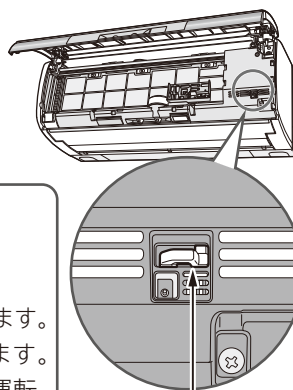
応急運転スイッチ
