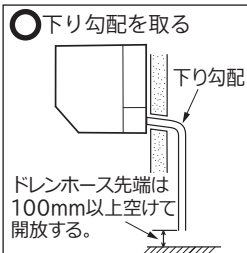
○下り勾配を取る
