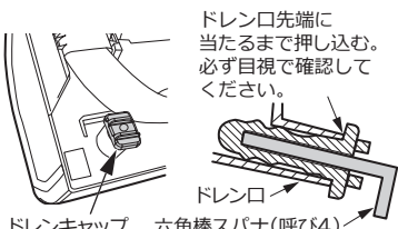
ドレン口 六角棒スパナ(呼び4) ドレンキャップ ドレンホース ドレンホース固定ねじ
