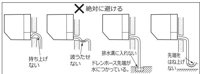
△絶対に避ける
