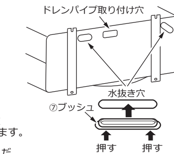
ドレンパイプ取り付け穴
