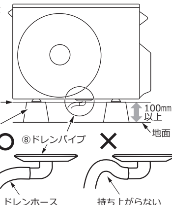
ドレンパイプ取り付け穴
