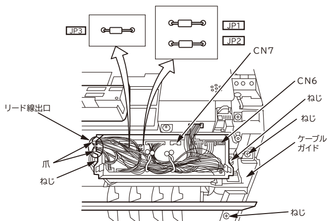
ジャンパー線部詳細
