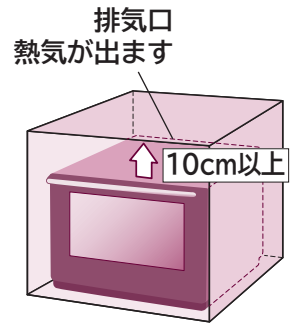
排気口 熱気が出ます 10cm以上 背面・側面は壁にぴったり 設置できます
