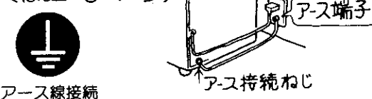
アース線接続
