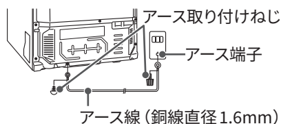
アース線(銅線直径1.6mm)
