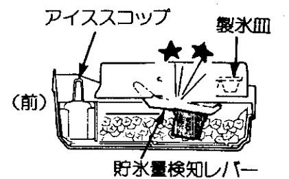
(前) 貯氷量検知レバー (自動製氷機のしくみについてはP19ページ)
