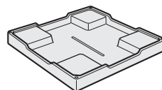
洗濯機用トレイ (YT-4) (幅640×奥行640×高さ83mm)
