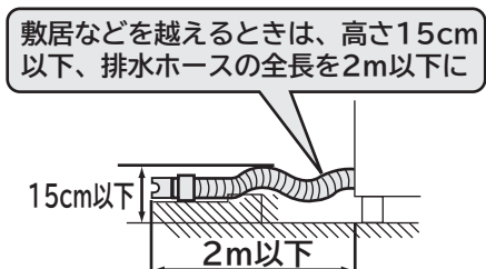
延長用排水ホースKW-50K1-023
