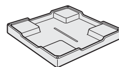
洗濯機用トレイ(YT-4) (幅640×奥行640×高さ83mm) 部品番号 YT-4-001
