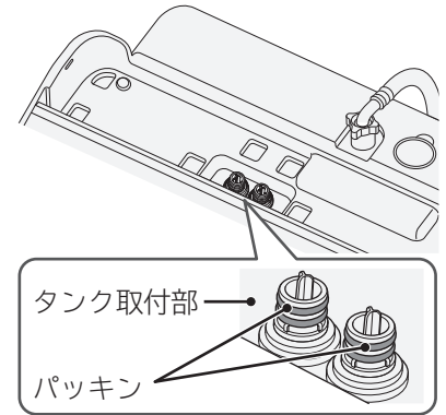
タンク背面図 (自動投入部ふたが取り付けられていない状態)
