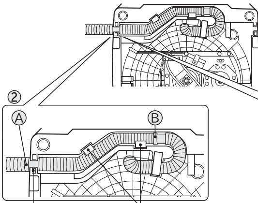
ホース引出口(右) ホースフック
