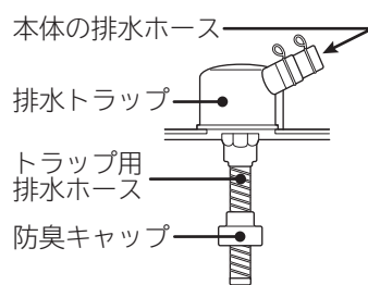
洗濯機排水トラップ (YT-T1)
