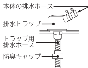
洗濯機用排水トラップ(YT-T1)
