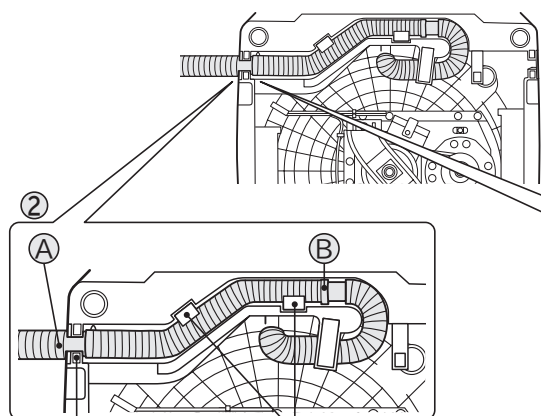
ホース引出口(右) ホースフック
