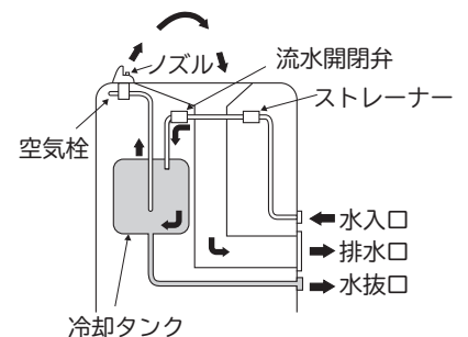
<水の流れ系統図>
