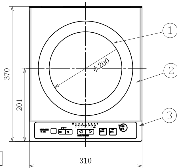
正面図
