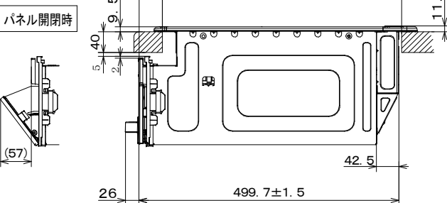
側面図
