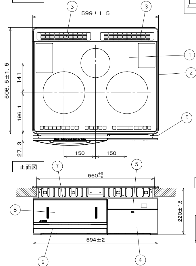
平面図
