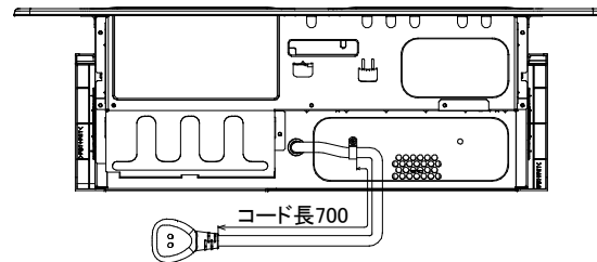
背面図
