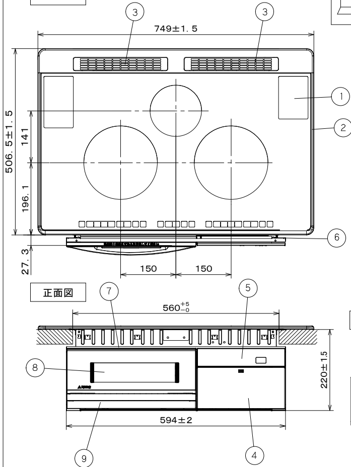
平面図
