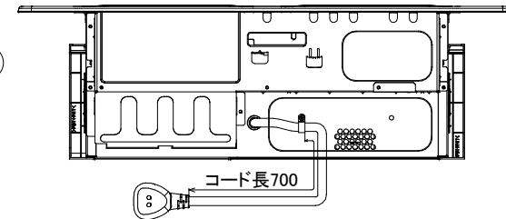
背面図
