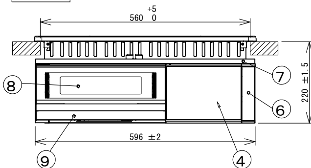
正面図
