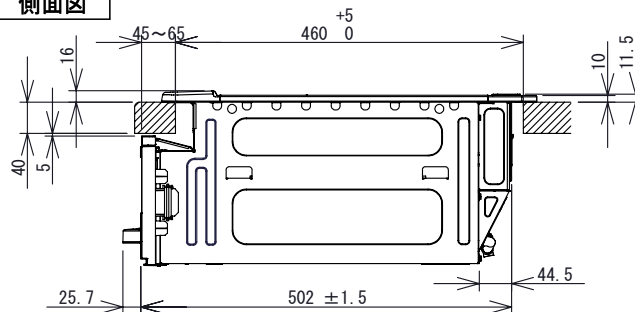
側面図
