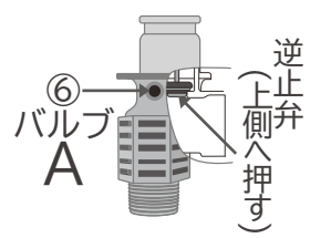
逆止弁位置(給水継手左視図)
