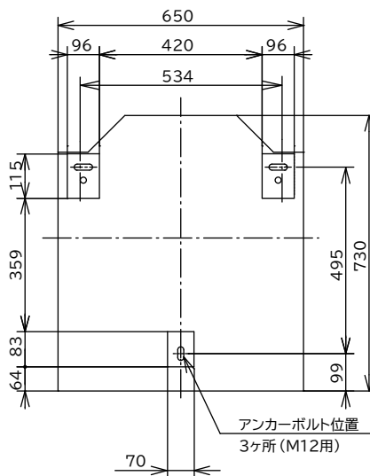
貯湯ユニット脚部寸法
