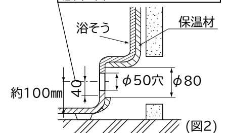
(図2) ベンチ部取付の場合
