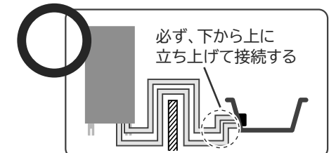
正しい施工例
