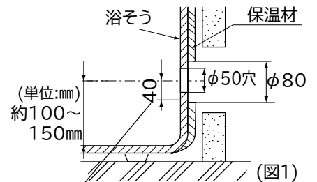
(図1) 穴の中心から40mm以内は底面の曲がりにかからないこと
