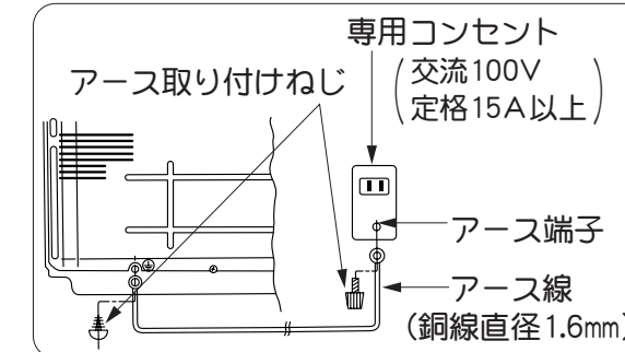
別売品：「アース線（2.5m）」 部品番号 NW-60R6 52
